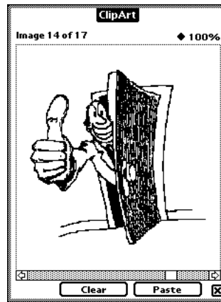
ClipArt Browser
