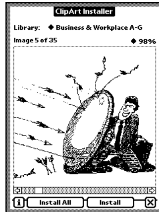
ClipArt Browser
